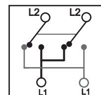
Moduł łącznika krzyżowego
